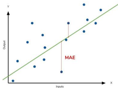
Gambar 6.4 Evaluasi menggunakan MAE
